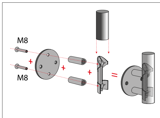
Contropiastra assemblata
