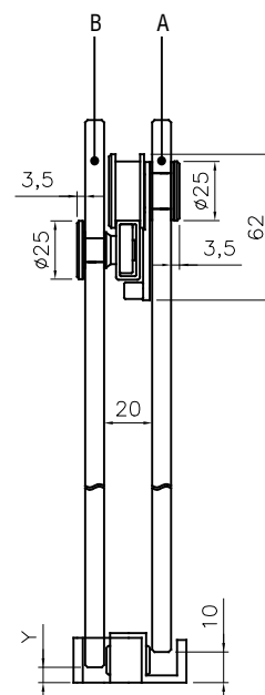
Vista in sezione section view
